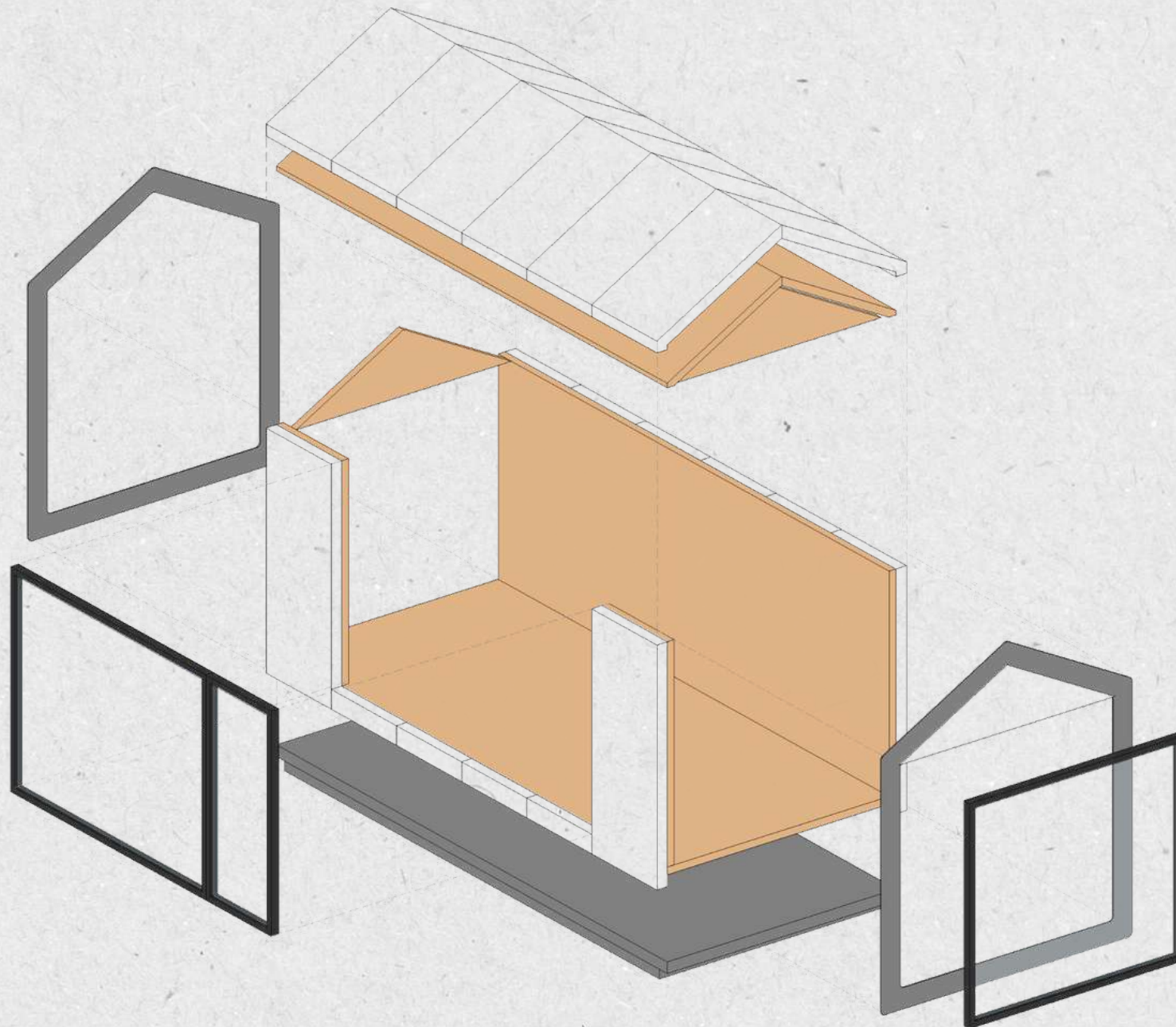
Modelado envolvente Minimal.
