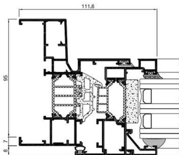
Sección acotada carpintería COR 70 OC Semivista RPT.
